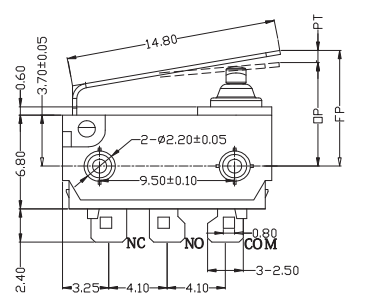
36# Lever
