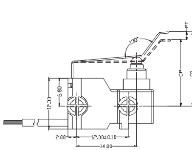
13# Lever
