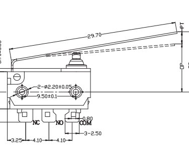
25# Lever
