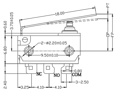
35# Lever
