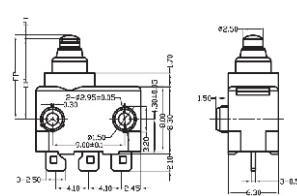
17 25 D1/D2 type left side posts
